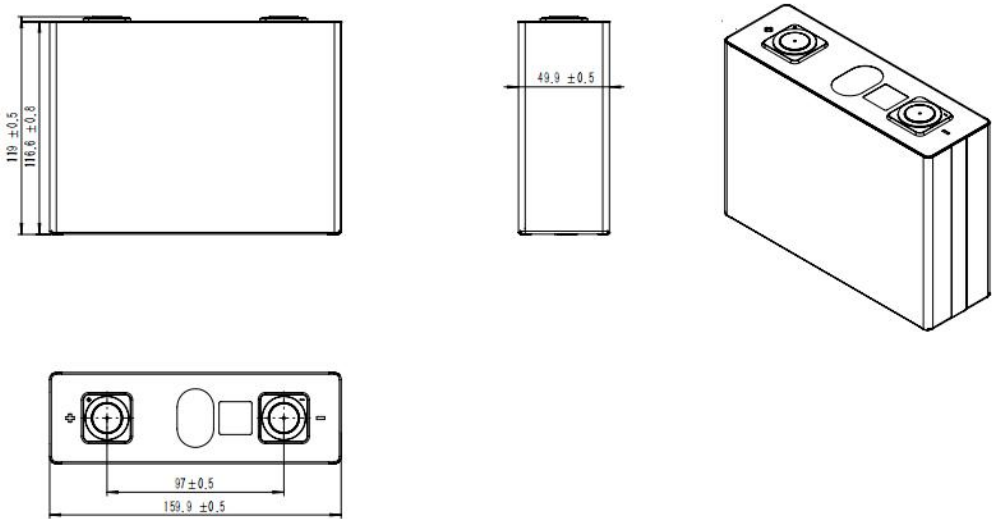
电芯的外观尺寸图
